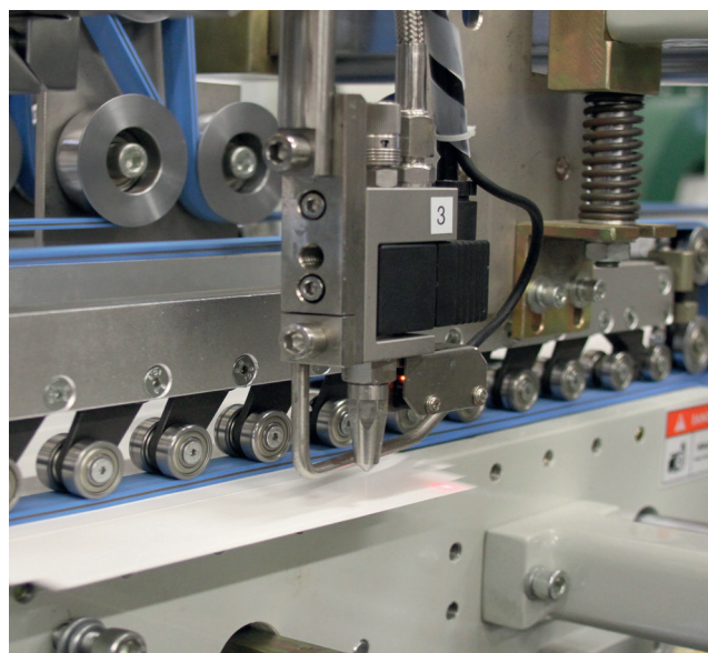
Leimdüsen mit Sensor
