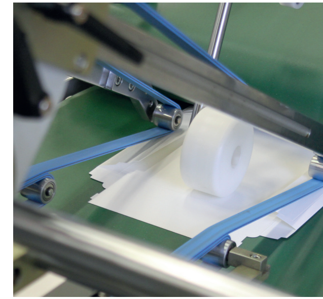
Zweispurklebung
